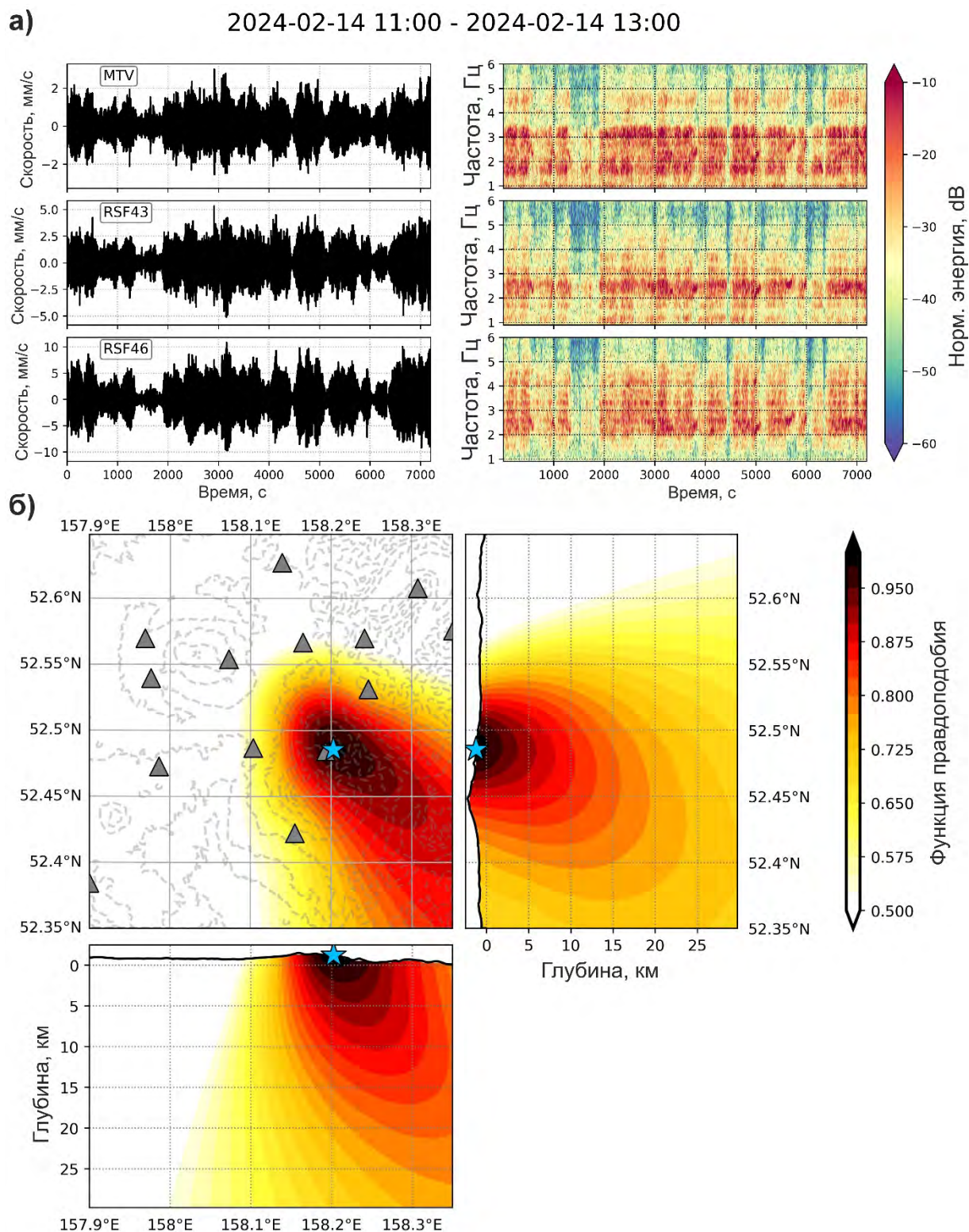
Рисунок 31. – Пример одной из наиболее когерентных двухчасовых записей тремора: а) – сигналы и спектрограммы; б) – соответствующее суммарное пространственное распределение вероятности локации источника сигнала.
