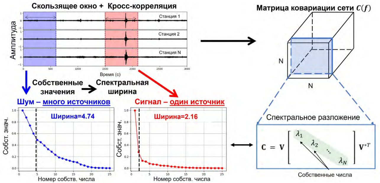
Рисунок 5. – Концептуальная схема процедуры оценки матрицы ковариации сейсмических записей и её спектральной ширины на примере записей, содержащих сильное землетрясение.
