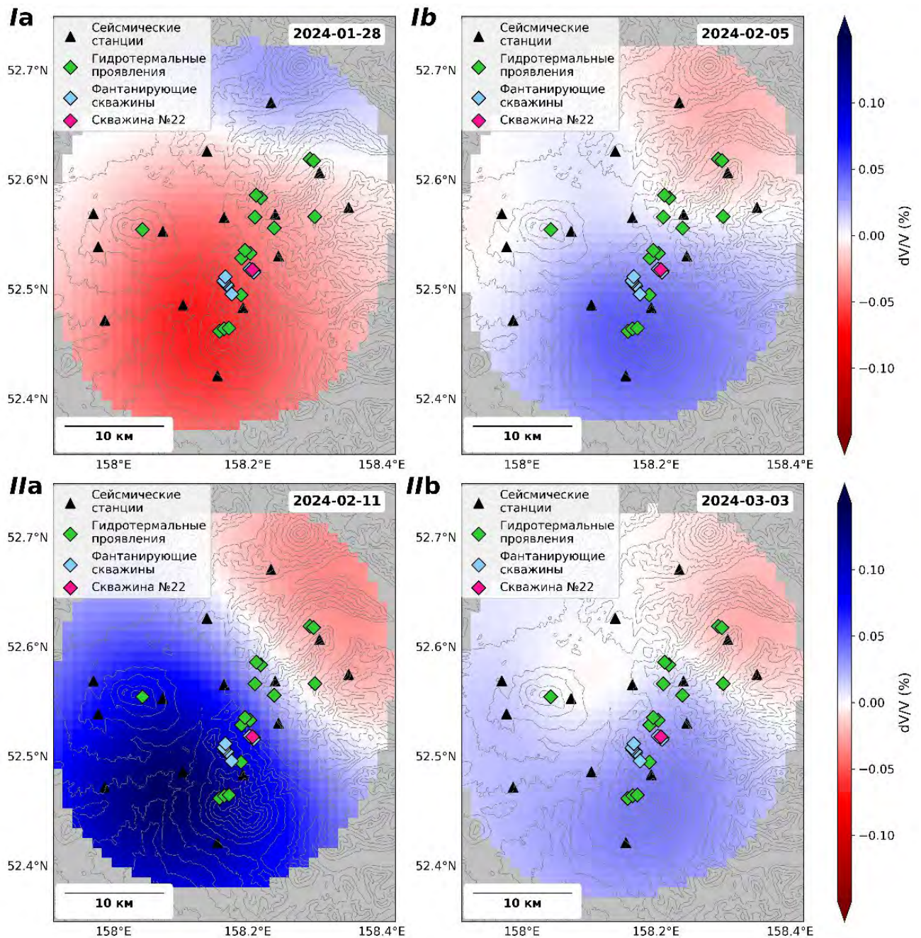
Рисунок 43. – Пространственные распределения вариаций скорости, рассчитанные для времени наблюдения Ia, Ib, IIa, IIb, отмеченные на рисунке 40. Изменения скорости отображены только для точек с индексом разрешения выше 0,7.
