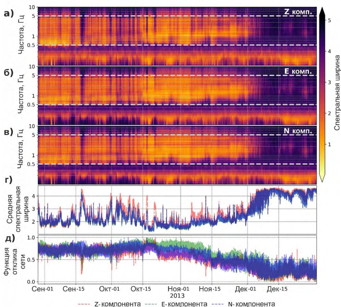
Рисунок 8. – Характеристика записанного волнового поля. На панелях а–с показана ковариационная матрица спектральной ширины, вычисленная для каждой частоты в течение 625-секундных перекрывающихся окон: а) Z-компонента, б) E-компонента и в) N-компонента. Две горизонтальные белые линии указывают целевую полосу пропускания для вычисления г) средней спектральной ширины и д) функции отклика сети.
