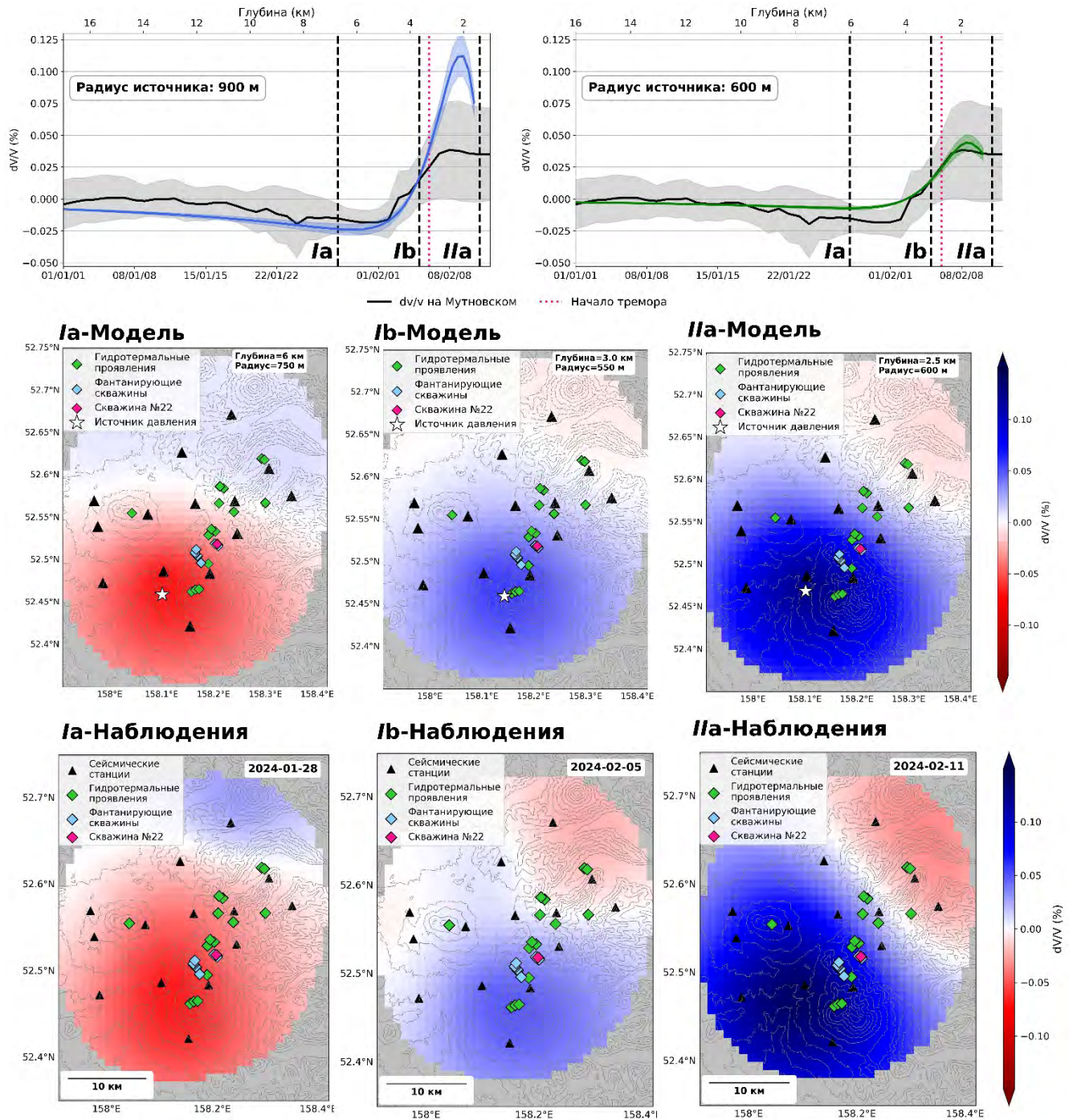
Рисунок 45. – Результаты синтетического моделирования изменений скоростей с использованием конечного сферического источника давления. В верхнем ряду показано сравнение среднего наблюдаемого значения dV/V в районе Мутновского геотермального поля (черная кривая) с результатами моделирования: левая и правая панели соответствуют источнику радиусом 900 м (синяя кривая) и 600 м (зеленая кривая), соответственно. В среднем ряду показаны синтетические карты пространственного распределения dV/V , соответствующие наблюдаемой карте, представленной в нижнем ряду. Ia, Ib и IIa соответствуют 28 января, 5 февраля и 11 февраля, соответственно.
