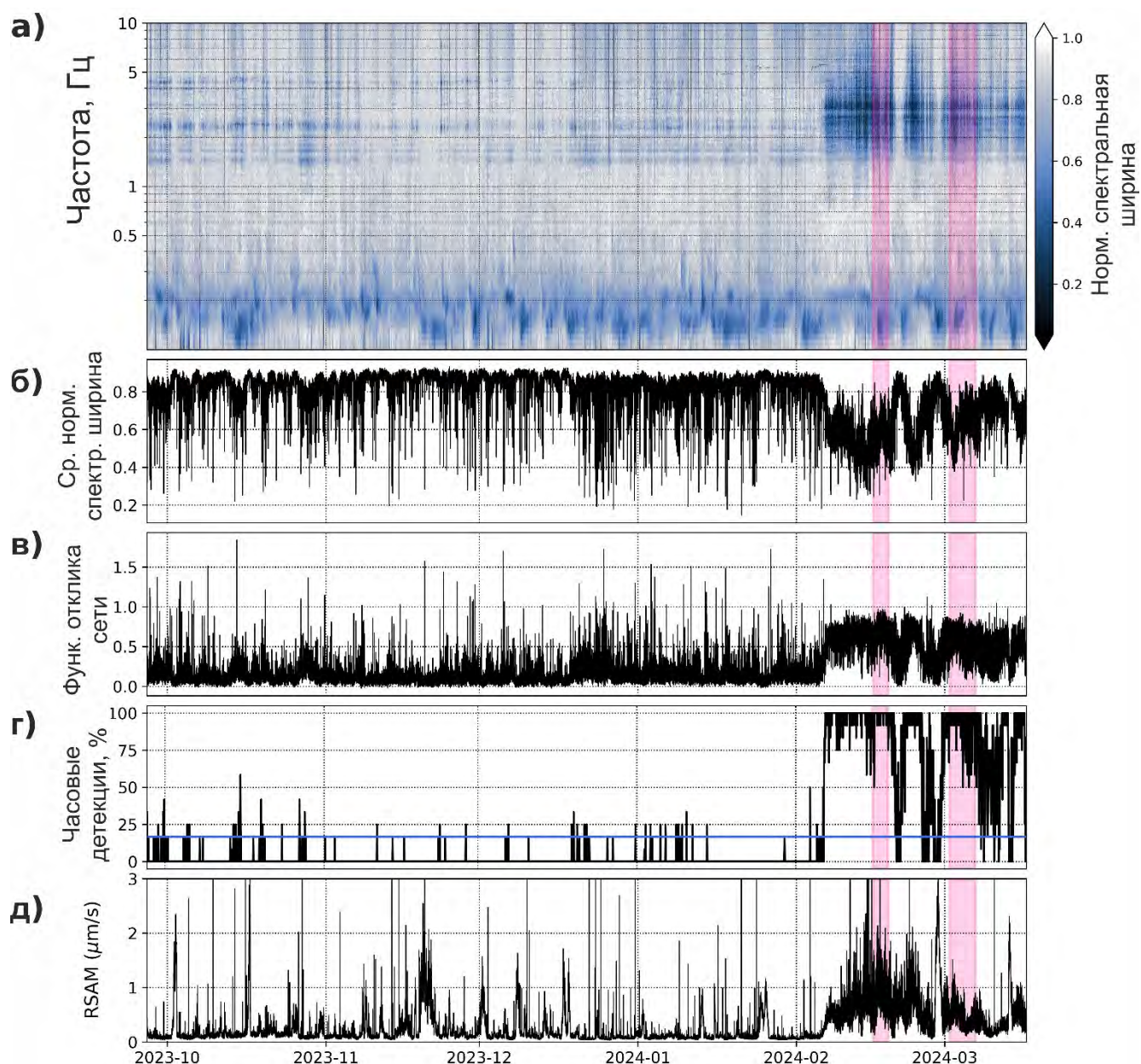
Рисунок 28. – Характеристика зарегистрированного волнового поля: (а) – спектральная ширина ковариационной матрицы, вычисленная для каждой частоты по 10-минутным перекрывающимся окнам; (б) – спектральная ширина, усредненная по частотному диапазону 1–5 Гц; (в) – отклика сети; (г) – процент обнаруженных окон, содержащих тремор, относительно почасовых записей (синяя линия указывает на одно обнаружение в час); (д) – RSAM для станции RSF46, вычисленная в частотном диапазоне 1–5 Гц с использованием 10-минутных окон. Розовые вертикальные полосы указывают на оценочное время гидротермальной активности.
