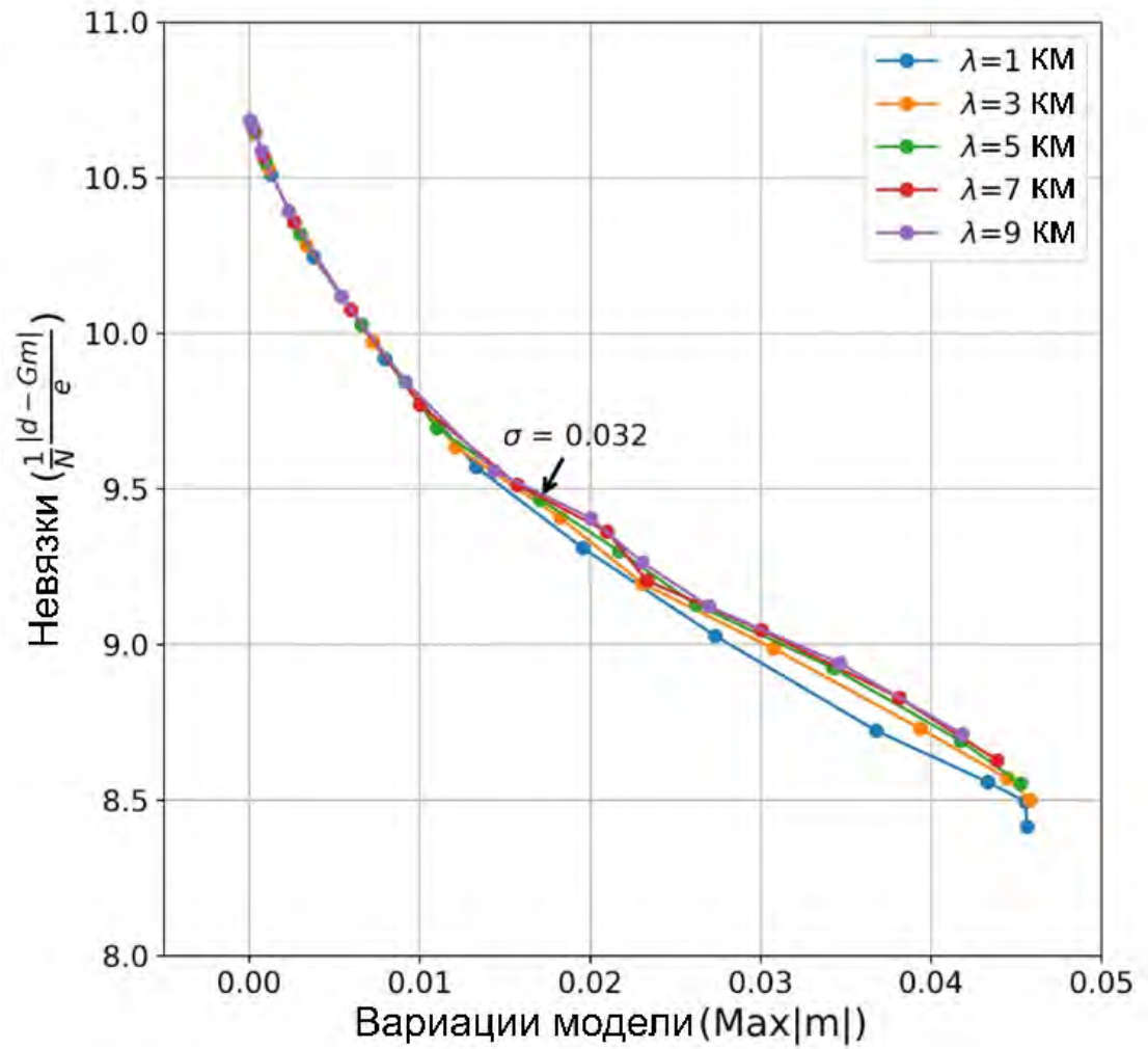
Рисунок 41. – L-кривая оценки пространственного распределения изменений скоростей. Черная стрелка указывает на использованные значения параметров регуляризации: \sigma = 0,032\% и \lambda = 5 км.
