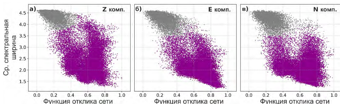
Рисунок 9. – Средняя спектральная ширина как функция от величины функции отклика сети. а) для Z-компоненты, б) для E-компоненты, в) для N-компоненты. Серым цветом обозначены наблюдения, классифицированные как фоновый шум. Фиолетовым цветом обозначены наблюдения, классифицированные как тремор.
