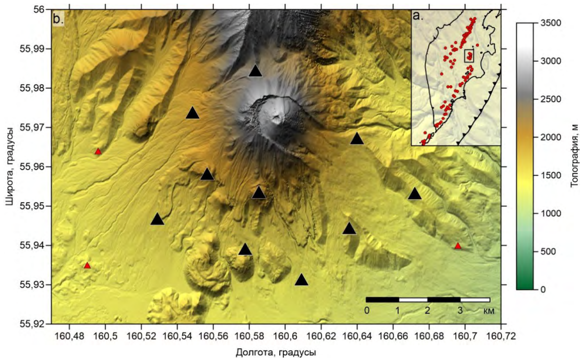
Рисунок 19. – Район исследования и конфигурация временной сети. а) Карта Камчатки с указанием района исследований (синий прямоугольник). Красные точки обозначают голоценовые вулканы. (б) Район исследований с отмеченными временными сейсмическими станциями (черные треугольники).
