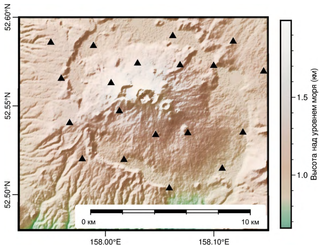
Рисунок 7. – Карта станций временной сейсмической сети, установленной на вулкане Горелый в 2013-2014 гг.
