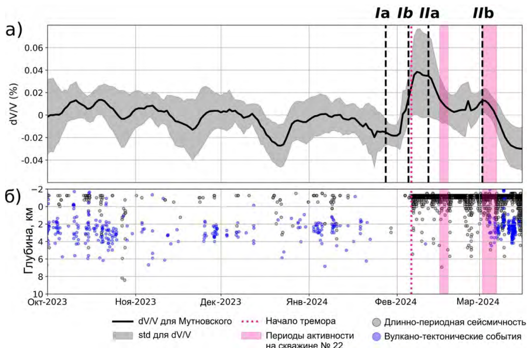
Рисунок 40. – Временные изменения сейсмических скоростей в окрестности Мутновского вулкана и Мутновского парогидротермального месторождения. а) Среднее значение и стандартное отклонение вариаций скорости с удаленным трендом для станций, расположенных рядом с вулканом Мутновский. Черные пунктирные линии обозначают выделенные этапы Ia, Ib, IIa и IIb. б) Глубинное распределение сейсмичности по данным КФ ФИЦ ЕГС РАН (вулкано-тектонические землетрясения) и гипоцентры длинно-периодной сейсмичности по результатам ковариационного анализа.
