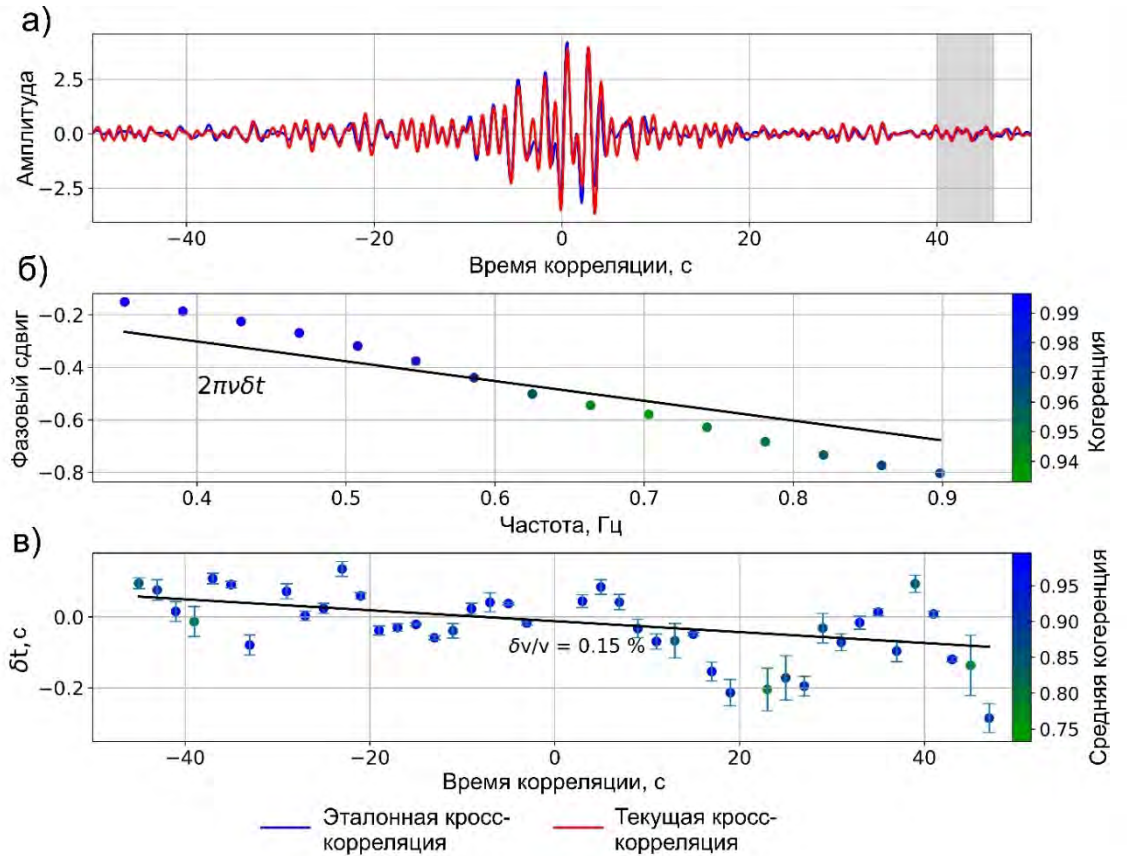
Рисунок 15. – Пример применения MWCS к кросс-корреляциям (между станциями BZ01-BZ02 в полосе пропускания 1–3 с на вулкане Безымянный) [Berezhnev et al., 2023]. (а) Синяя кривая – эталонная кросс-корреляция, полученная как среднее значение за период с 1 сентября по 1 ноября. Красная кривая – суточная кросс-корреляция за 17 ноября 2017 г. (б) Фазовые сдвиги между эталонной и суточной кросс-корреляциями в области, выделенной цветом на рисунке (а). Черная линия – тренд, полученный с помощью взвешенной линейной регрессии фазовых сдвигов. (в) Полученный временной сдвиг в зависимости от времени корреляции. Черная линия – тренд, указывающий на относительные изменения скорости.
