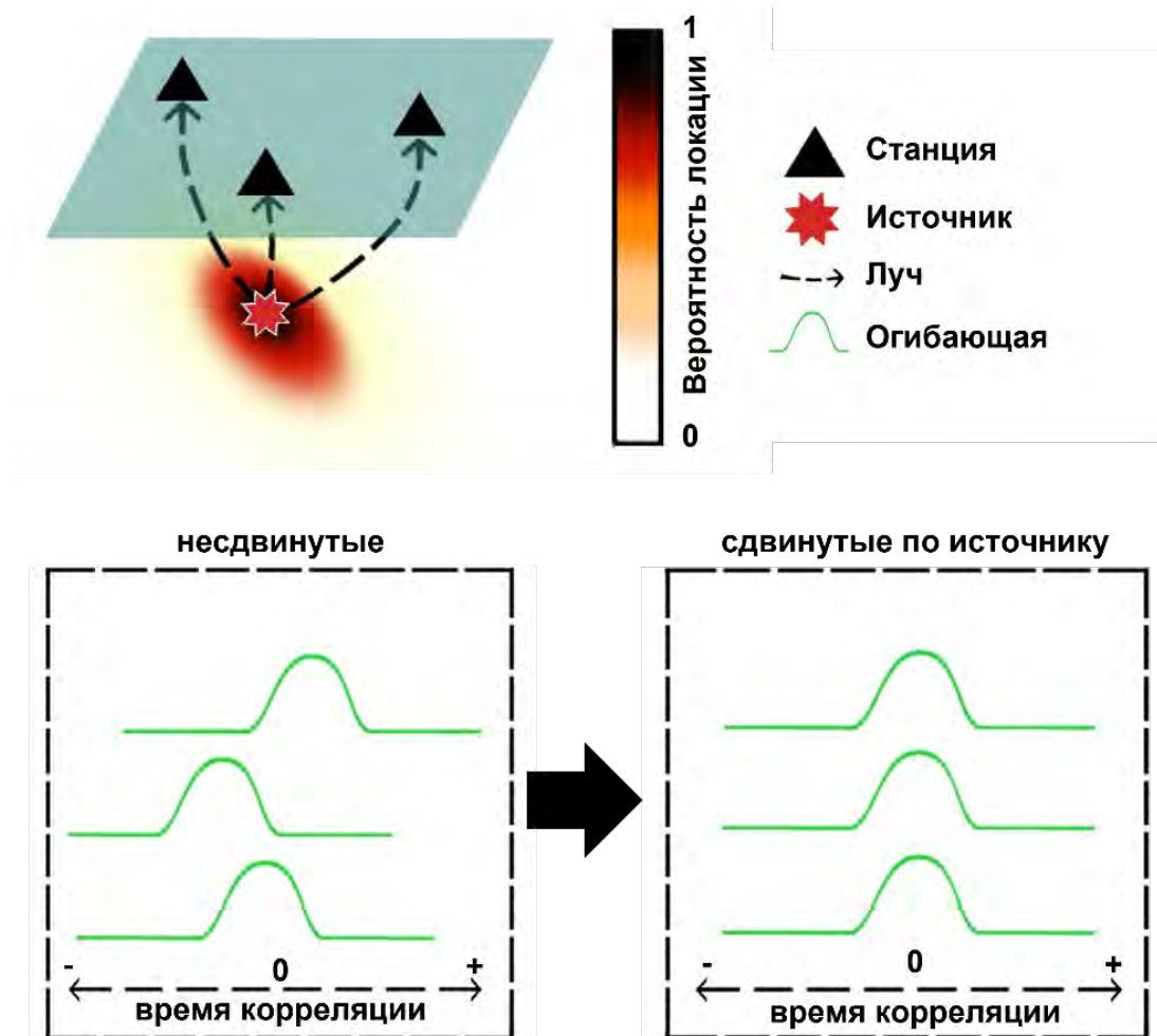
Рисунок 6. – Концептуальная схема процедуры локации источника сигнала на примере сигнала на рис. 5.
