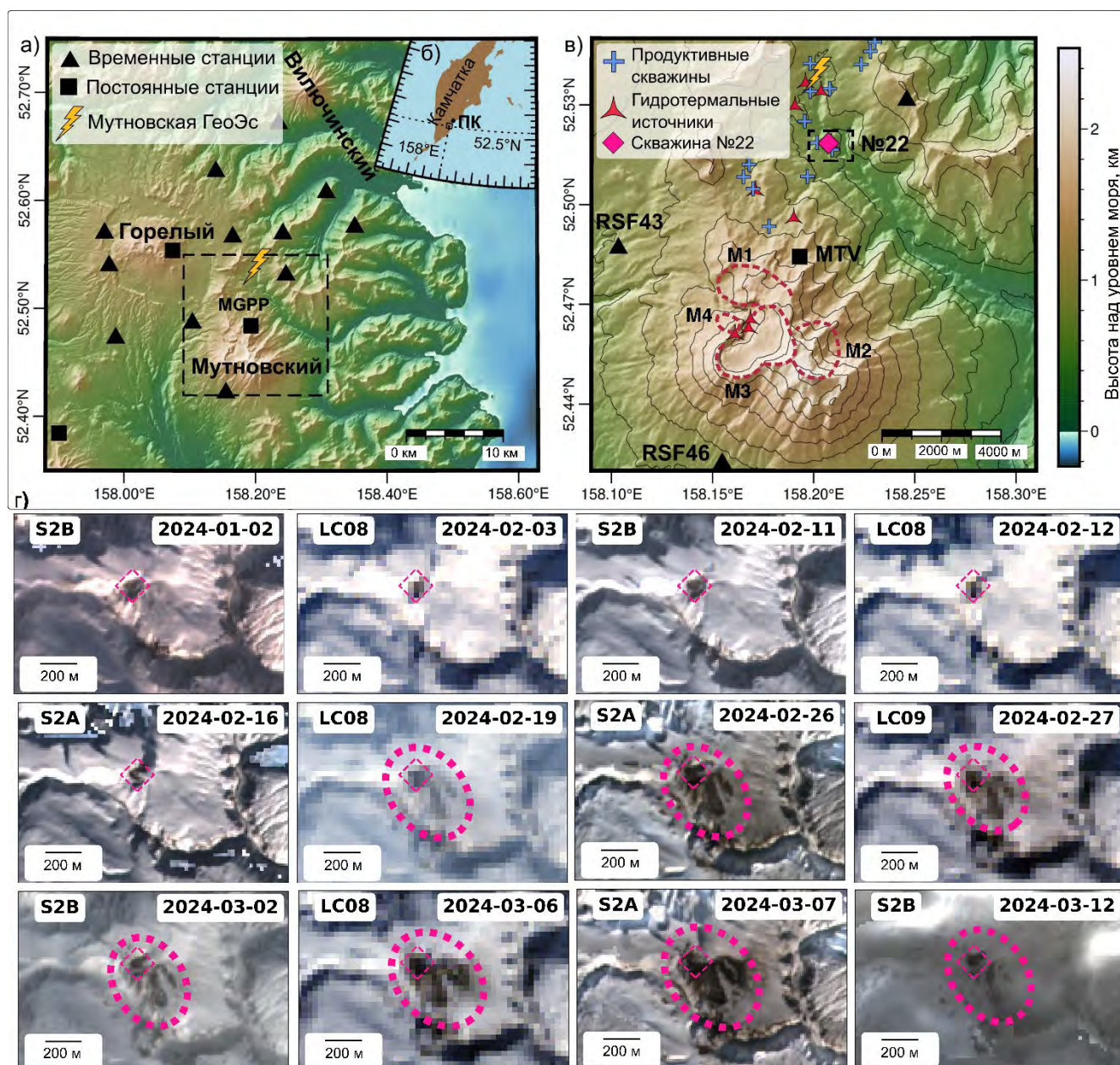
Рисунок 26. – Карта (а) исследуемого региона с указанными сейсмическими станциями, использованными для анализа, с (б) врезкой географического расположения и (в) увеличенным изображением Мутновского вулкана и района геотермальной электростанции (черный пунктирный квадрат на панели а). ПК — Петропавловск-Камчатский, М1-М4 – центры вулканической активности Мутновского. (г) Спутниковые снимки места геотермальной активности за период наблюдений (черный пунктирный прямоугольник на панели в). Район скважины № 22 выделен розовым пунктирным ромбом. Розовый эллипс выделяет область, затронутую геотермальной активизацией. Код спутника указан в левом углу каждого изображения (Sentinel-2A/2B как S2A и S2B; Landsat-8/9 как LC08 и LC09), а дата съемки указана в правом углу.
