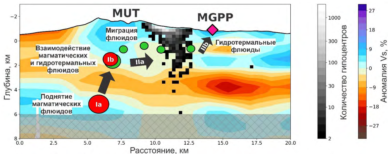
Рисунок 47. – Концептуальная модель процессов в магма-гидротермальной системе вулкана Мутновский во время его активизации в начале 2024 г. Красными кругами отмечены источники давления, связанные с восходящими магматическими флюидами, а зелеными – источники давления, связанные с гидротермальными флюидами. Розовым ромбом обозначена скважина №22. MUT – Мутновский вулкан, MGPP – Мутновская геотермальная электростанция. На фоне изображено вертикальное сечение аномалии скорости поперечных волн, которое было модифицировано из Belovezhets et al., [2026], серая заштрихованная область обозначает зону низкого разрешения томографической модели. Распределение гипоцентров тремора изображено черно-белым градиентом цвета.
