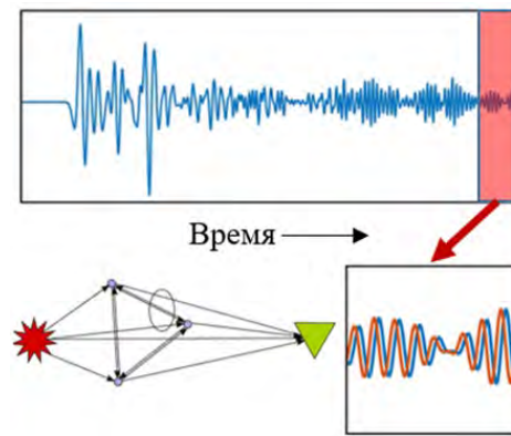
Рисунок 14. – Иллюстрация отклика кода-волны на изменения скорости в среде. Зеленый треугольник – приёмник, красная звезда – источник, фиолетовые точки – рассеиватели, черные стрелки – пути распространения волны, овалом отмечен участок с возмущением скорости, синий график – кода волны до возмущения, красный – после возмущения [Singh et al., 2019].
