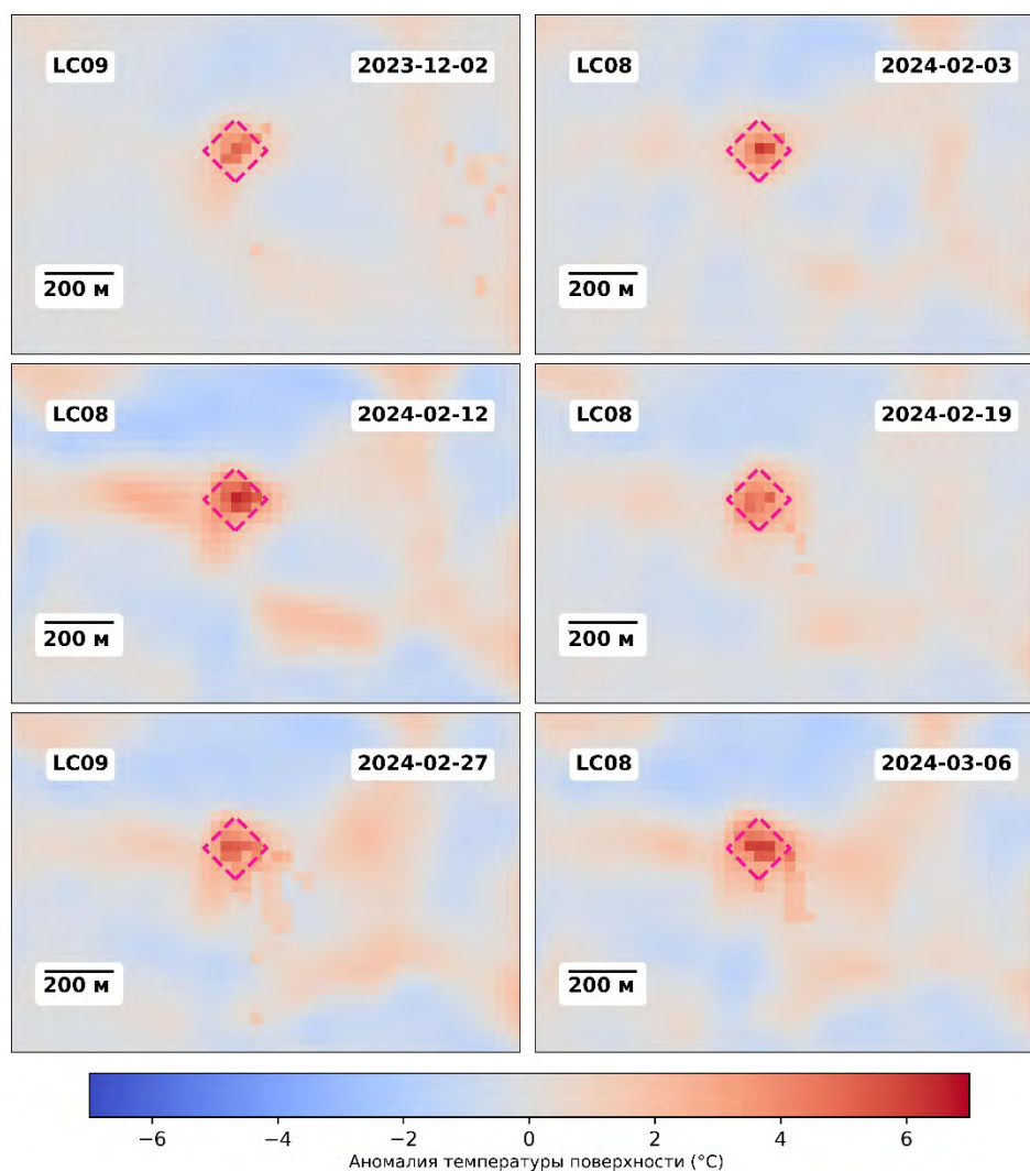
Рисунок 27. – Аномалия температуры поверхности около скважины №22 за период наблюдений. Аномалия определяется как отклонение от фоновой температуры, вычисленной как температуры поверхности земли, сглаженная гауссовым окном шириной 1 км. Область скважины № 22 выделена розовым пунктирным ромбом. Код спутника указан в левом углу каждого изображения (Landsat-8/9 как LC08 и LC09, соответственно), дата изображений указана в правом углу.
