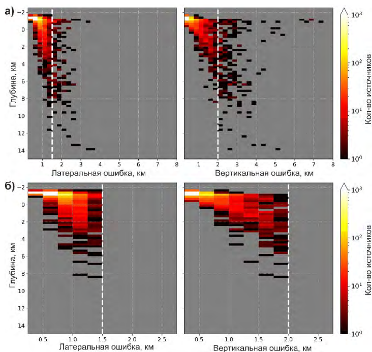
Рисунок 33 а) – Распределение неопределенностей местоположения источника по глубине, который оценивается как среднее расстояние от максимумов распределения функционала локации до изоповерхности величины 99% от максимумов. б) – Распределение по глубине неопределенностей местоположения источника после удаления местоположений с высокой неопределенностью. Белая пунктирная линия указывает пороговое значение.
