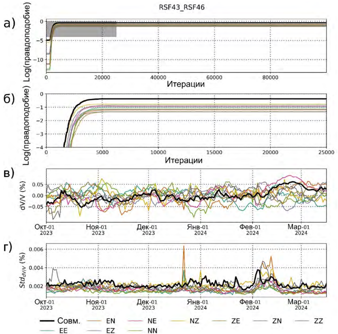
Рисунок 37. – Пример инверсии методом Монте-Карло цепей Маркова для оценки изменений скорости. Черная кривая показывает результаты, основанные на измерениях, полученных с помощью предложенного подхода MWCS с совместным использованием всех компонент, а цветные кривые - результаты, основанные на измерениях, полученных с помощью однокомпонентного подхода MWCS. На панели а) показана логарифмическая функция правдоподобия в течение фазы отжига. На панелях б) и в) показаны среднее значение и стандартное отклонение апостериорного распределения, соответственно.
