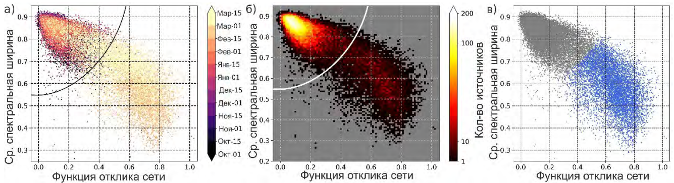
Рисунок 30. – Классификация сейсмического волнового поля на сигнал-шум. NRF как функция от средней нормированной спектральной ширины. а) – характеристика записей от времени наблюдения; б) – гистограмма характеристик сигналов; в) – полученная классификация исследуемых записей: серый цвет обозначает наблюдение, классифицированное как фоновый шум, синий цвет обозначает наблюдение, классифицированное как тремор. Черные (а) и белые (б) эллипсы представляют собой разделение между сигналами шума и сигналом тремора. Эллипс задан положением центра (x_0, y_0) = (0.13, 0.94) , большой и малой полуосями a, b = 0.35, 0.5 и углом поворота \phi = -\pi/3 .
