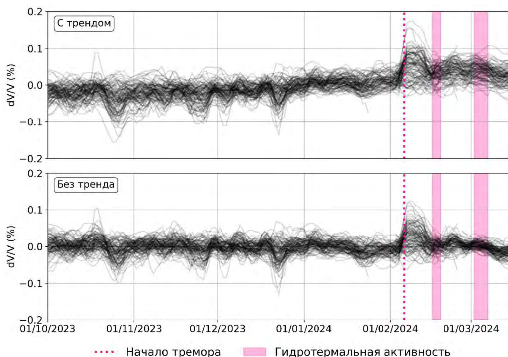
Рисунок 38. – Полученные временные ряды изменений скорости. На верхней панели показаны исходные временные ряды; на нижней панели – временные ряды после процедуры удаления тренда.
