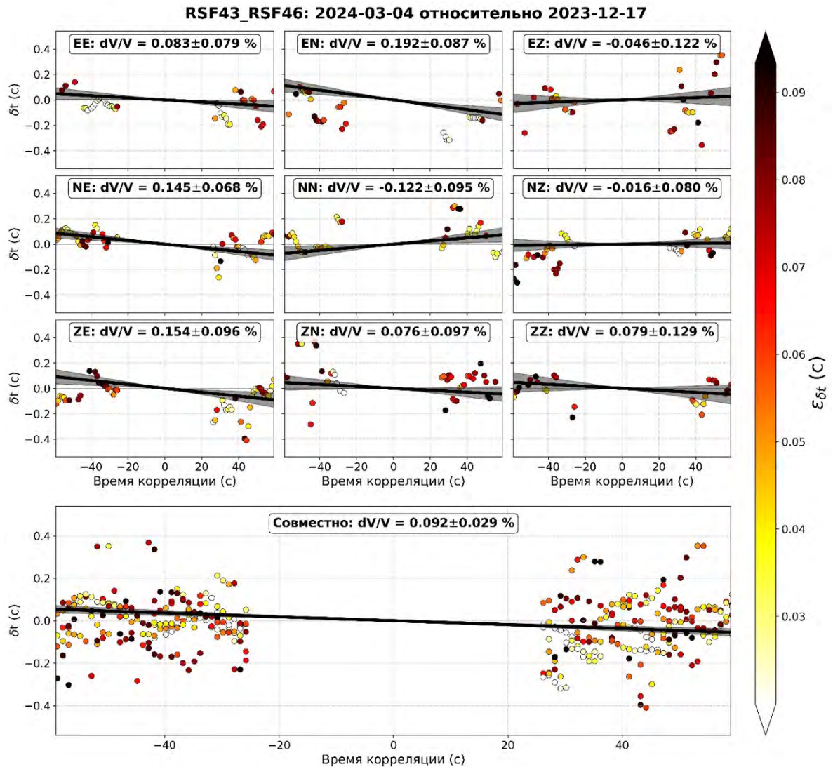
Рисунок 16. – Пример оценок JC-MWCS для кросс-корреляций пары станций (на примере станций RSF43 и RSF46 на вулкане Мутновский). Компоненты тензора кросс-корреляции и соответствующие им оценки изменения скоростей и их неопределенности отмечены в верхней части каждого графика.
