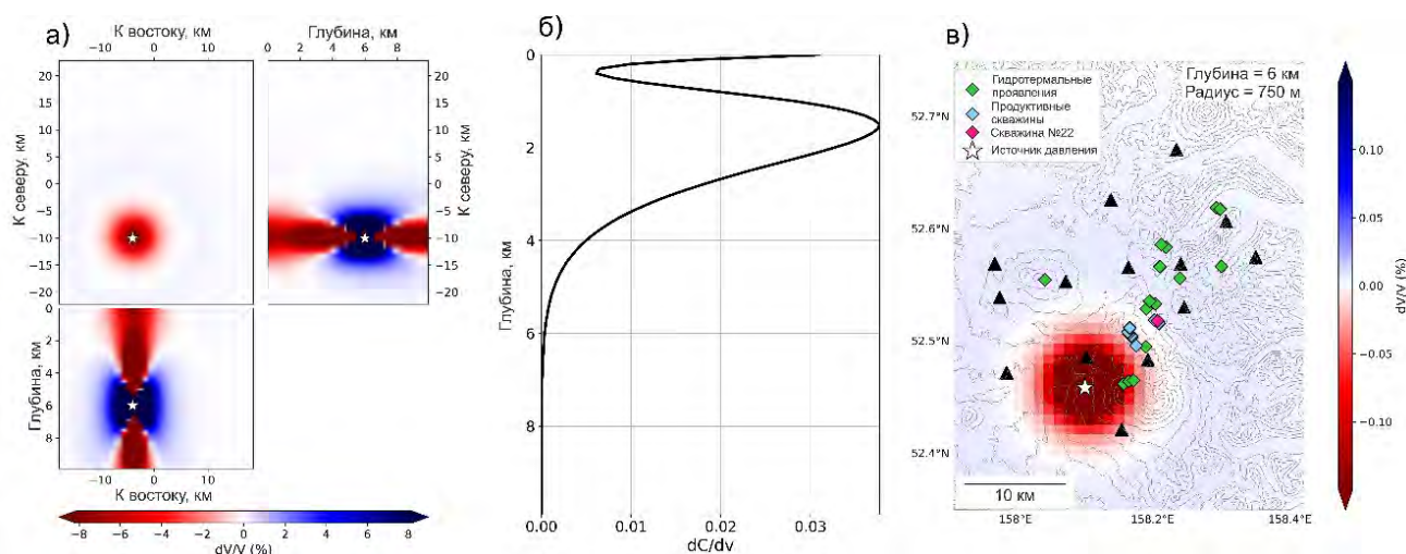
Рисунок 44. Результаты моделирования dV/V с помощью сферического источника конечного давления. Панель а) – трехмерное распределение вариаций скорости, вызванных источником радиусом 760 м, центр которого отмечен звездой. Панель б) – ядро чувствительности фазовой скорости волны Рэлея для центрального периода целевого частотного диапазона (2 с для полосы пропускания 1-3 с), оцененное в одномерной скоростной модели [Belovezhets et al., 2026] в) – карта смоделированного пространственного распределения изменений скорости.
