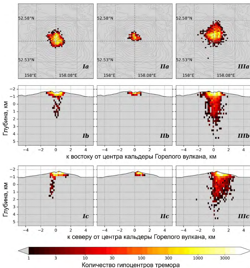
Рисунок 11. – Гистограммы гипоцентров источников тремора для кластеров I, II и III. Пересечение серых пунктирных линий на рисунках верхнего ряда указывает на центр кальдеры вулкана Горелый. Верхний ряд (Ia, IIa, IIIa) показывает суммарную гистограмму, спроецированную на поверхность. Средний ряд (Ib, IIb, IIIb) отображает суммарную гистограмму, спроецированную на сечение «восток-запад», а нижний ряд (Ic, IIc, IIIc) представляет те же данные, спроецированные на сечение «север-юг».
