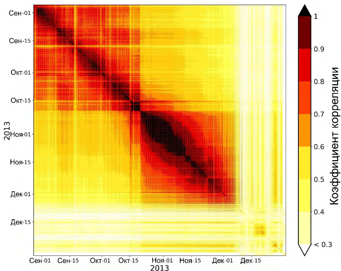
Рисунок 10. – Усредненная по компонентам матрица корреляции между первыми собственными векторами всех проанализированных ковариационных матриц.
