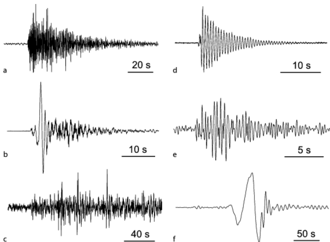
Рисунок 4. – Пример классификации сеймовулканических сигналов. а) – Вулкано-тектоническое землетрясение, произошедшее между островами Миякедзима и Кодзудзима, Япония; б) – Взрывное землетрясение, наблюдавшееся на вулкане Асама, Япония; в) – Тремор на вулкане Фудзияма, Япония; д) – Длинно-периодное событие, зафиксированное на вулкане Кусацу – Ширане, Япония; е) – Длинно-периодное событие, наблюдавшееся на вулкане Гуагуа-Пичинча, Эквадор; ф) – Очень длинно-периодное событие, произошедшее под островом Миякедзима, Япония (отфильтровано фильтром высоких частот выше 0.05 Гц) [Kumagai, 2009].
